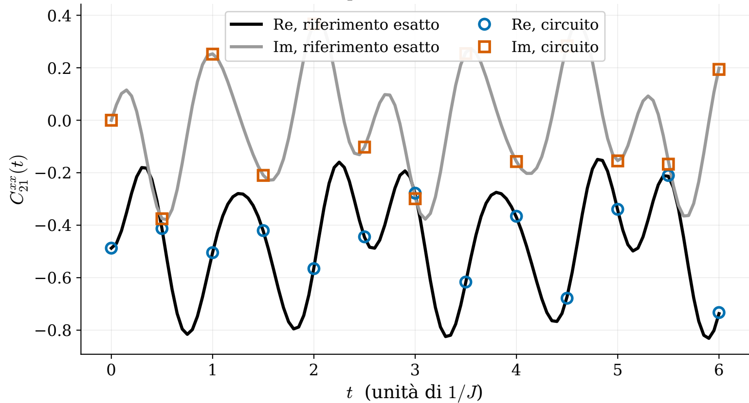
Il circuito con l'ancilla riproduce il calcolo classico (Scenario A)
